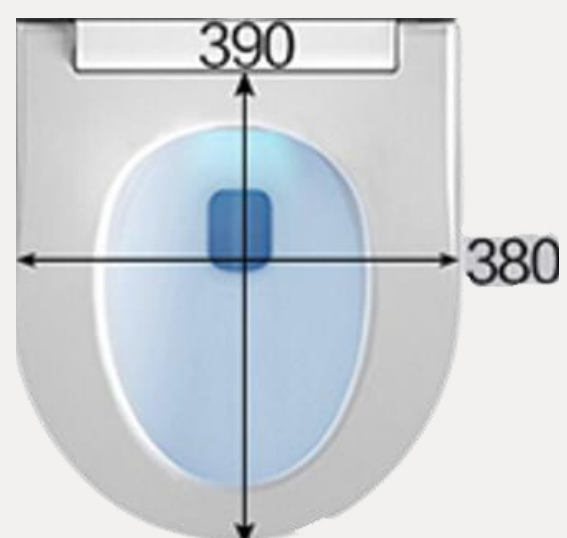
Medidas interiores y exteriores del asiento (en mm).
